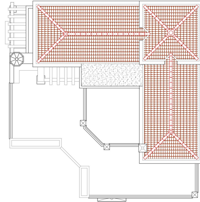
PLANTA CUBIERTAS
