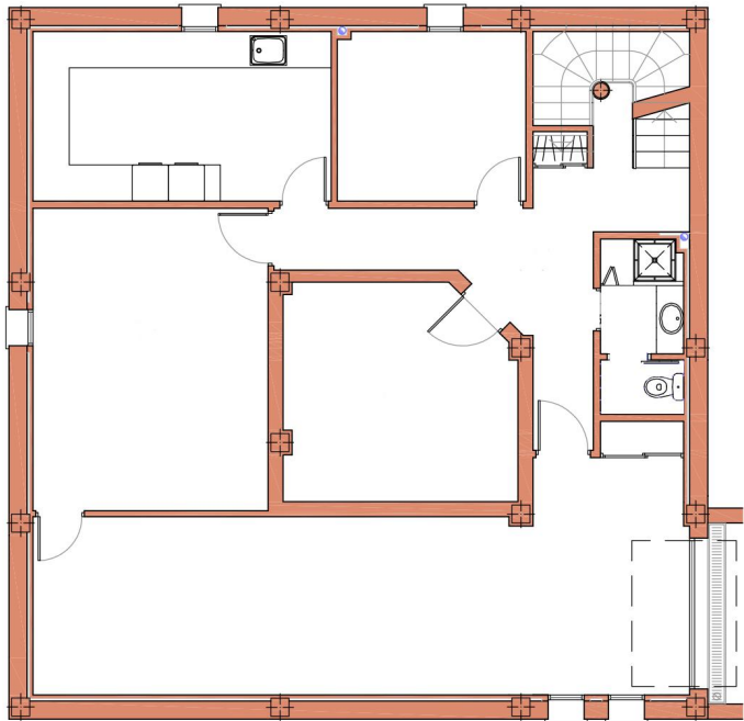
PLANTA GARAJE
